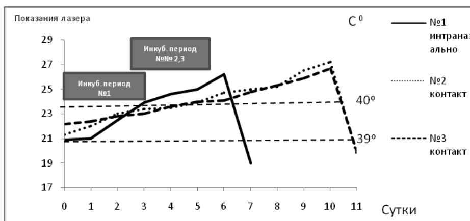
Рис. 2 Результаты измерения температуры тела у диких свиней (группа №2), инфицированных изолятом № 161/23 вируса АЧС (№1 – интраназальное и пероральное введение вируса, № 2,3 – контактное заражение).
